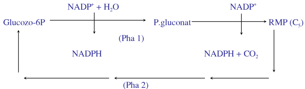
Hình 4.4. Sơ đồ vận tất của chu trình pentozophosphat
